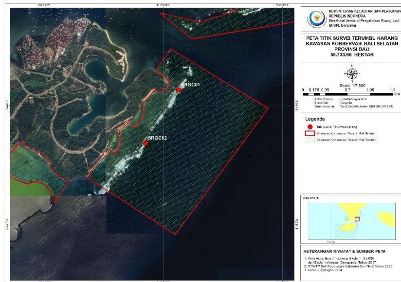
Gambar 8. Peta Lokasi Pengambilan Data Terumbu Karang
